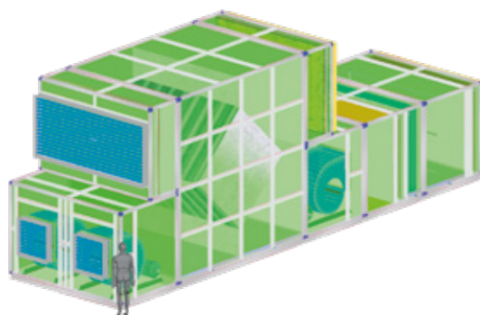
14 Standardgrößen mit einer Förderleistung von 1500 m³/h bis 128000 m³/h
