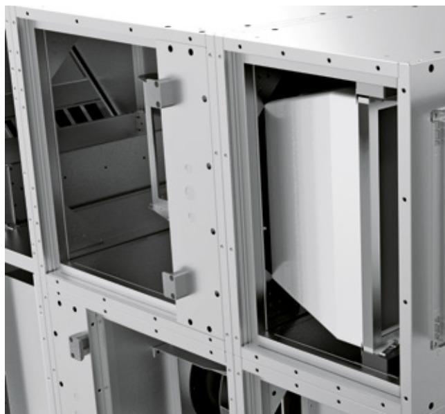
PVC-Profilsystem im Gehäuse der Anlage
