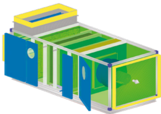
Einteiliger Aufbau
